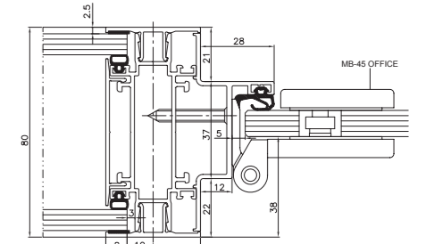
Door - horizontal view
