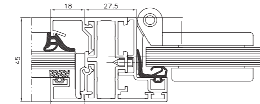
Door stud – section view
